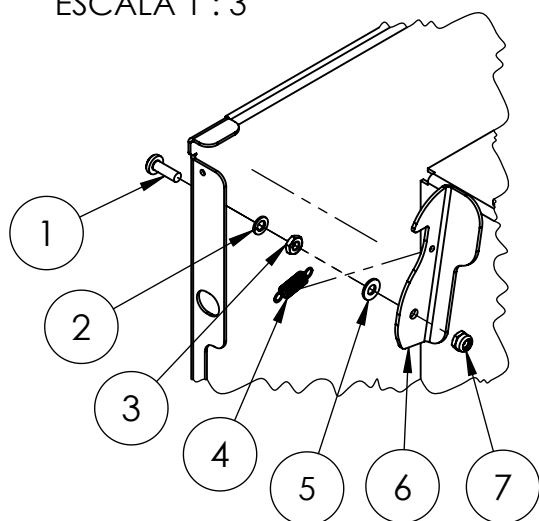
DETALHE A ESCALA 1 : 3
